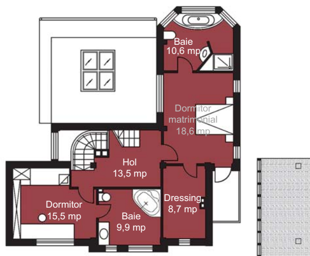
PLAN ETAJ
