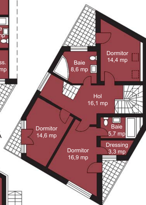
PLAN ETAJ
